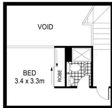
LOFT
